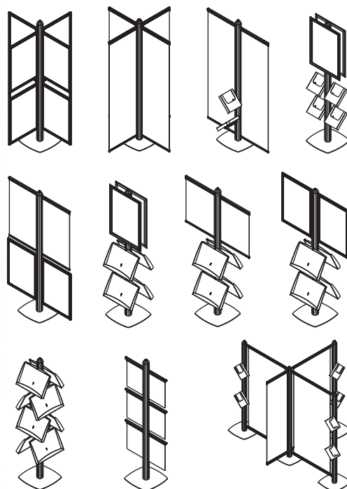
Some possible variations using 4 channel profile Variationen bei 4 Kanälen
