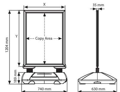
WindPro tool UYUP480945
