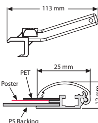
Levertool / Öffnungsapparat ARTICLE: UYUP047000
